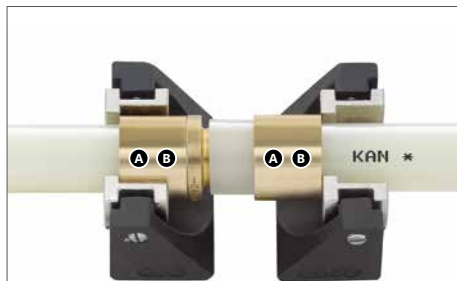
Монтаж двухсторонних соединителей (с другой стороны) Ø12×2, Ø14×2, Ø18×2, Ø18×2,5
